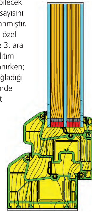
Pencere Isı Aktış Diyagramı Uf:1,07 W/m² °K Uw: 0,93 W/m² °K
