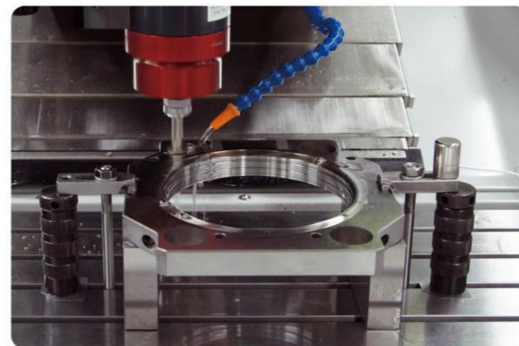
精密模具件加工 High precision mold
