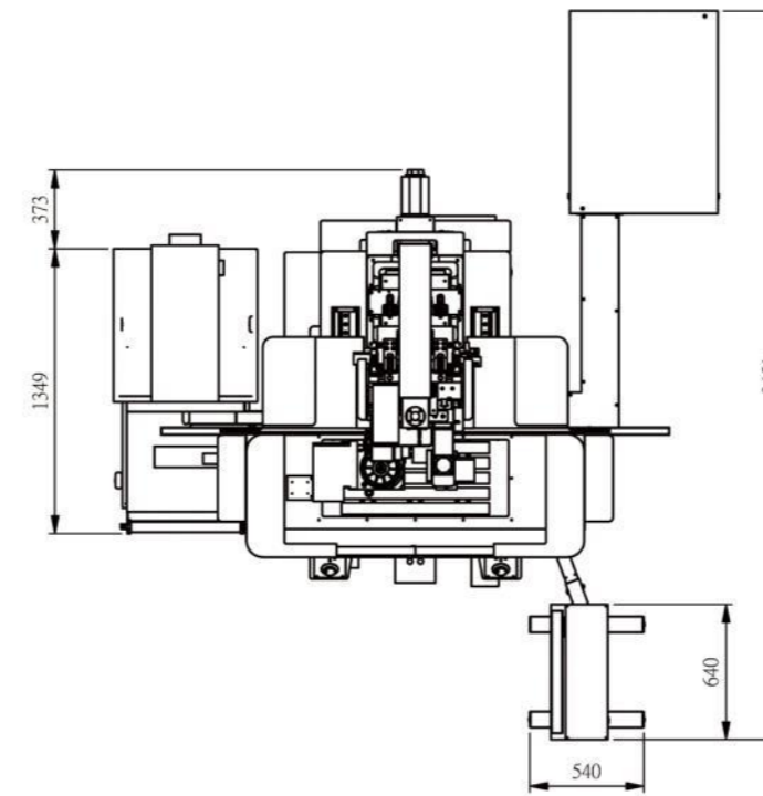
JG-510GC 外齒輪研磨機
