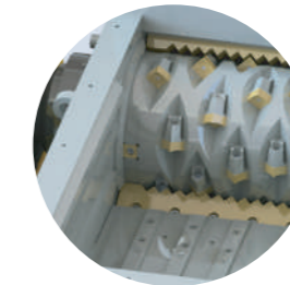
Parçalama Rotoru
