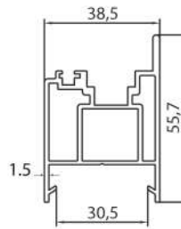
AURA ESPAGNOLETTE LOCK PROFILE 112
