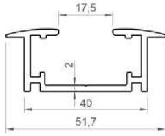
EŞİKSİZ KASA PROFİL 103
