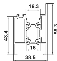
AURA-PLUS ESPAGNOLETTE LOCK PROFILE 212
