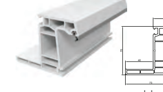
PERVAZLI KASA PROFİLİ
