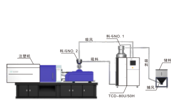
1对1 二段送料示意图(标准) 1To1 2-stage diagram
