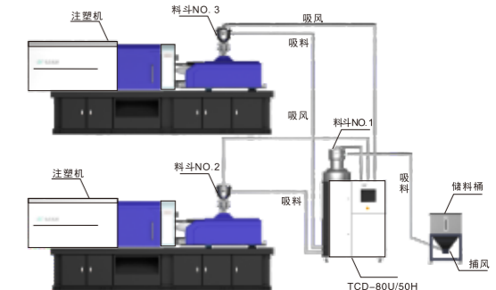
1对2 三段送料示意图(标准) 1To2 3-stage diagram
