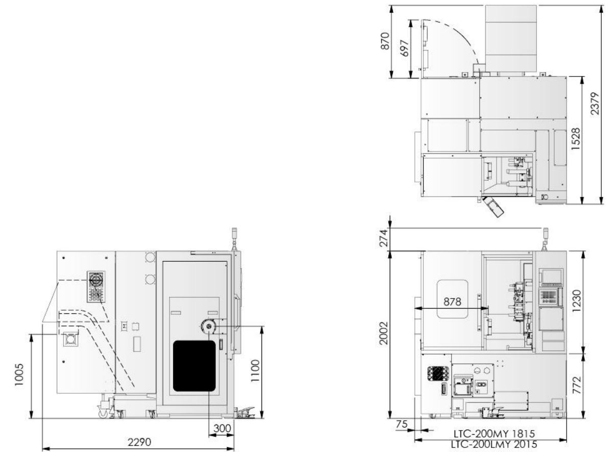
LTC-200MY/LTC-200LMY
