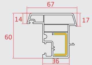
HARAİETLİ ORTA KAYIT (Overhung Profile)
