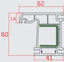
KASA (Frame Profile)
