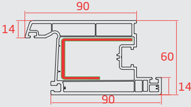
İÇE AÇILIR KAPI (Door Sash Profile)
