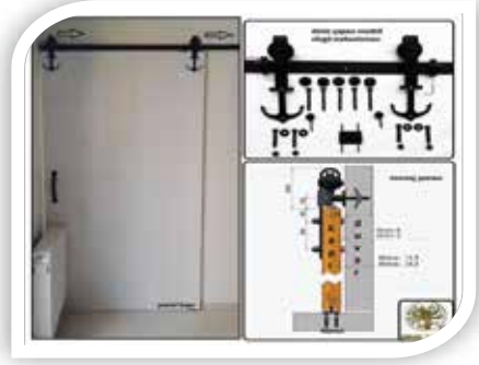
AT NALI MODELİ TEK KAPI SÜRGÜ MEKANİZMASI
