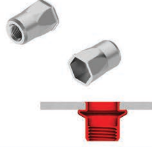
Inox Yarım Altı köşe Sıfır Kafa Inox Half - Hex. Reduced Head
