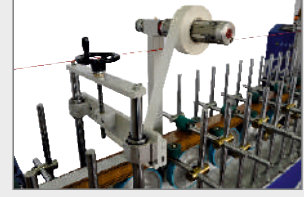
KORUYUCU BANT KAPLAMA İSTASYONU PROTECTIVE TAPE WRAPPING STATION УЗЕЛ НАНЕСЕНИЯ ЗАЩИТНОЙ ПЛЕНКИ
