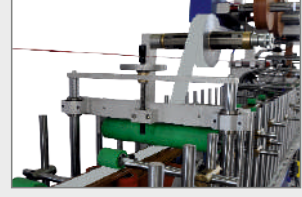
ÇİFT YÜZEY KORUYUCU BANT KAPLAMA İSTASYONU DOUBLE SURFACE PROTECTIVE TAPE LAMINATION STATION ДВУХСТОРОННЯЯ СИСТЕМА РАЗМОТКИ И НАНЕСЕНИЯ ЗАЩИТНОЙ ПЛЕНКИ
